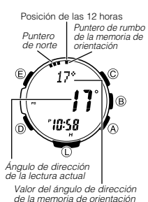
Valor del ángulo de dirección de la memoria de orientación
