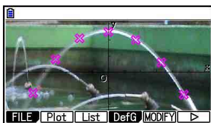
Pisteiden piirtäminen
