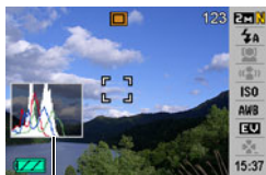
直方图
