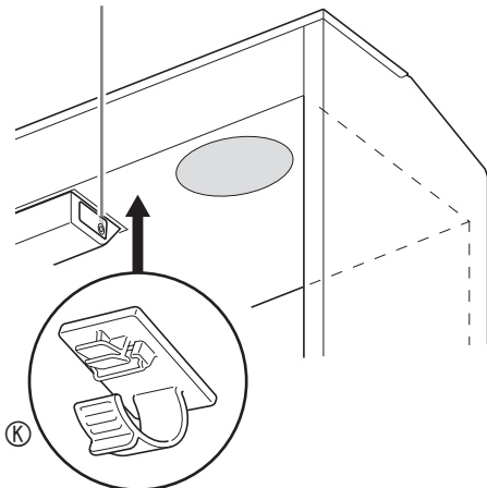
DC 12V-Anschluss
