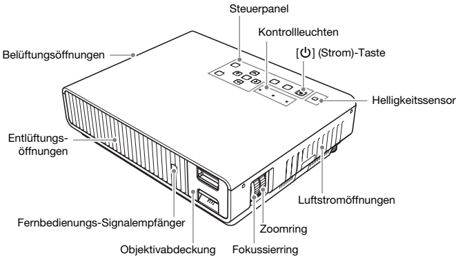
Projektionsobjektiv
