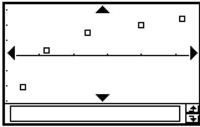
Streudiagramm
