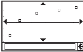
Streudiagramm
