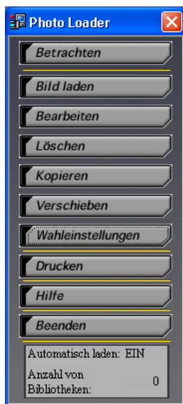
Photo Loader Funktions-Schaltflächen
